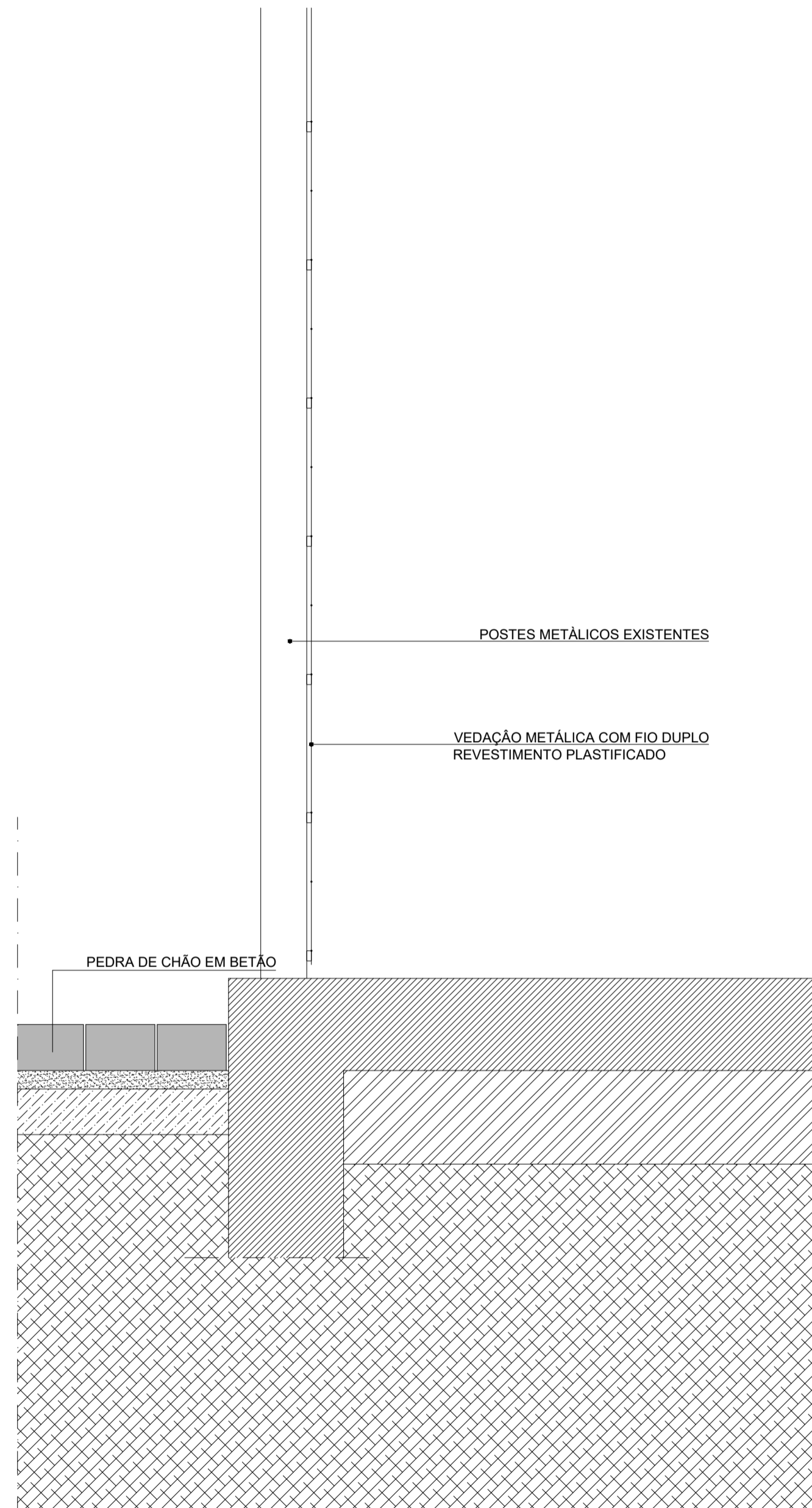
PORMENOR P02
